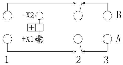
JQX-2010M
