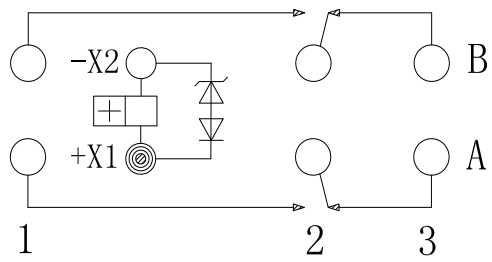
JQX-2110M
