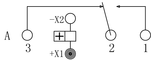
JQC-1010M
